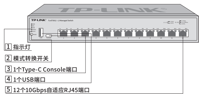
图1-2 TL-ST5012前面板示意图
