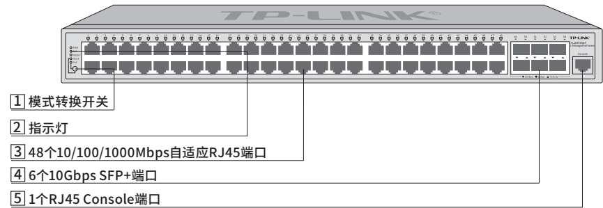
图1-4 TL-SH5654P/TL-SH5654PE前面板示意图
