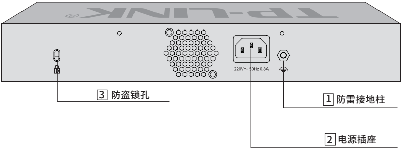
图1-7 后面板示意图
