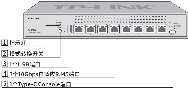
图1-3 TL-ST5008前面板示意图
