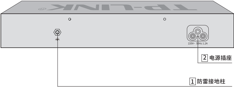
图1-6 后面板示意图
